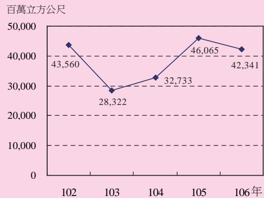
圖 2.2.2.2 各區水庫進水量
