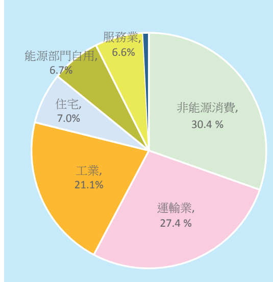
圖 2.2.1.3 106 年次級能源之國內消費
