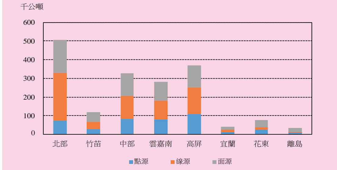
圖 2.1.1.6 106年空氣污染排放量－空品區與污染源
