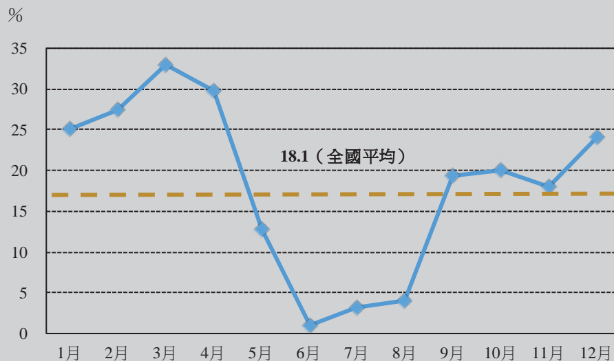
圖 2.1.1.7 106 年 AQI>100 之站日數比率
