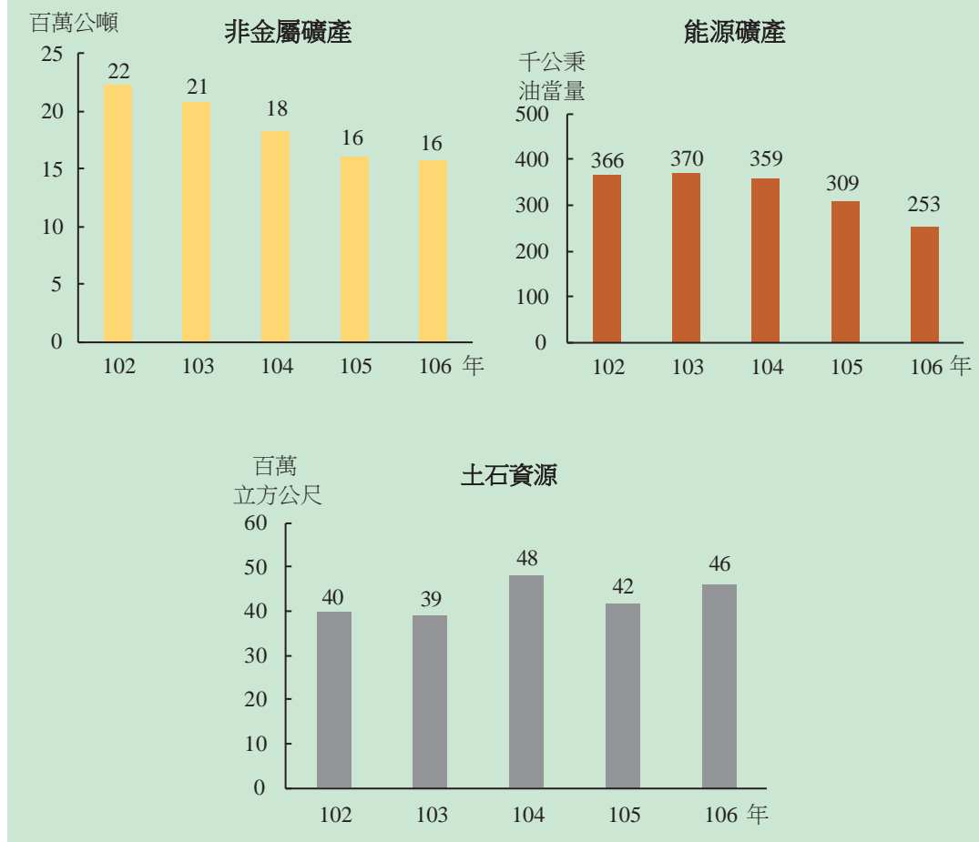
圖 1.5 礦產及土石資源開採量
