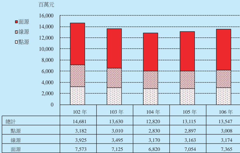
圖 2.1.1.9 空氣品質質損值
