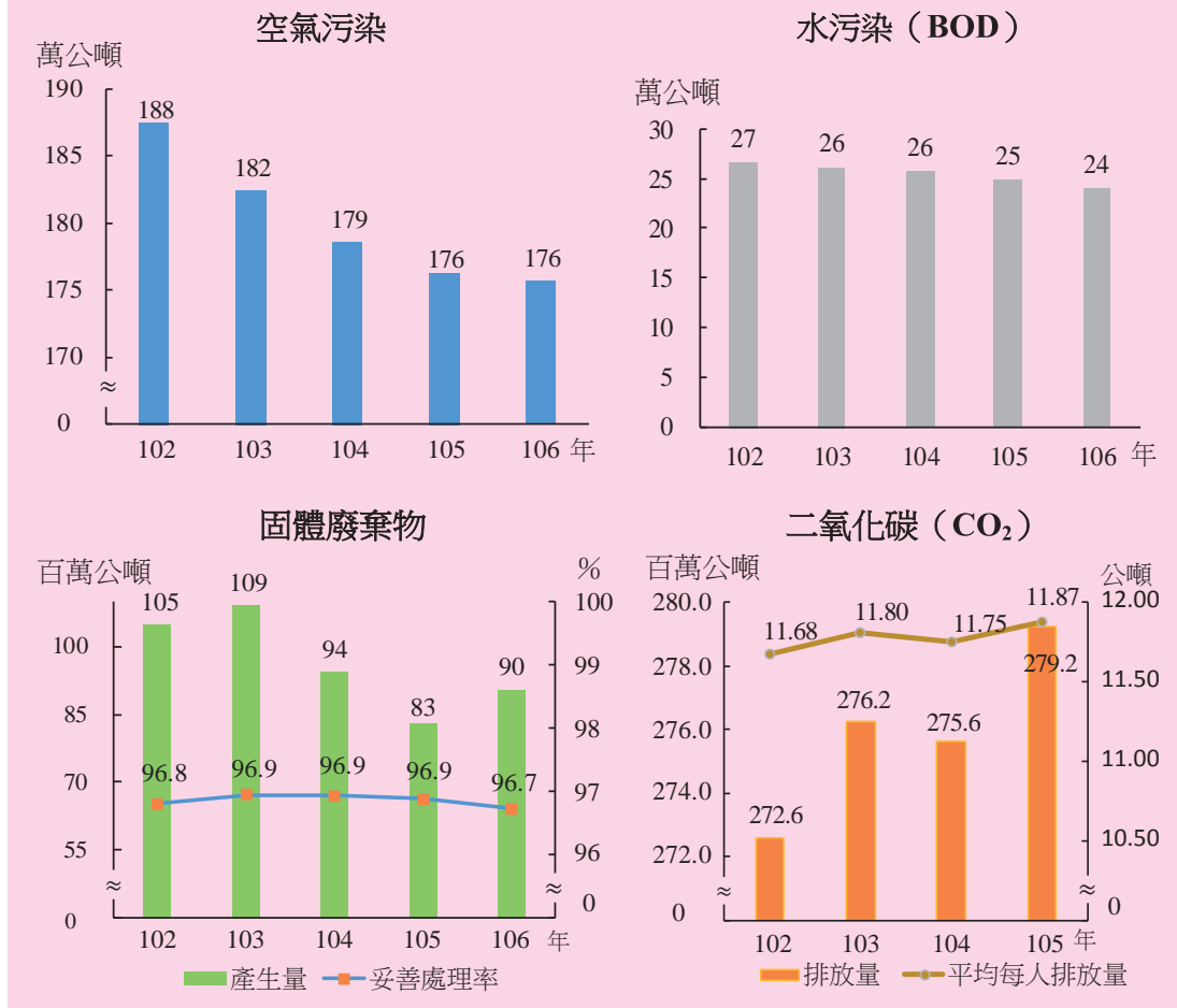
圖 1.1 污染物排放量
