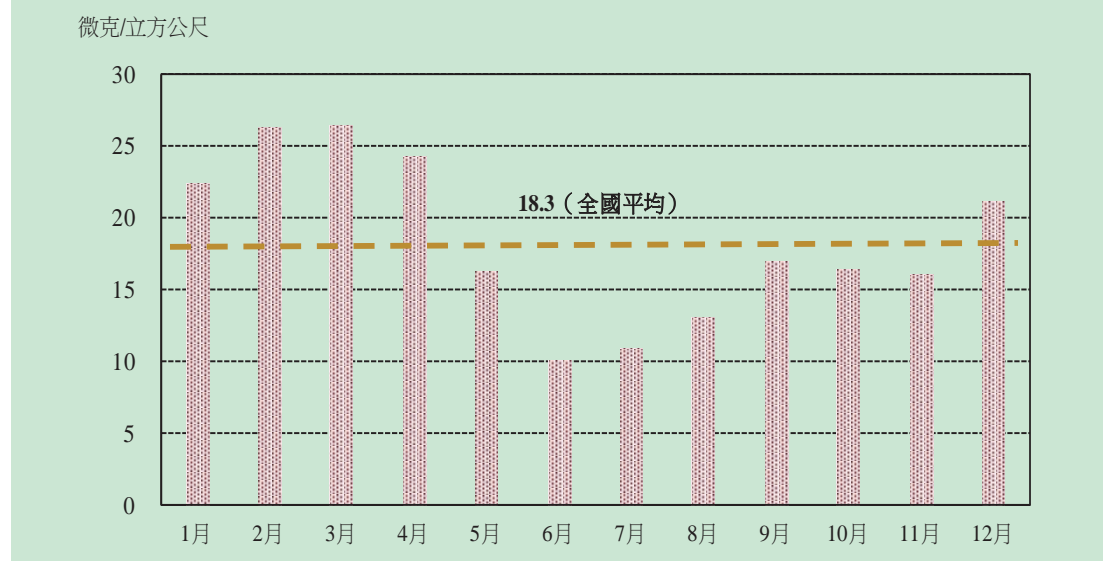
圖 2.1.1.8 106 年細懸浮微粒 (PM 2.5 ) 濃度值
